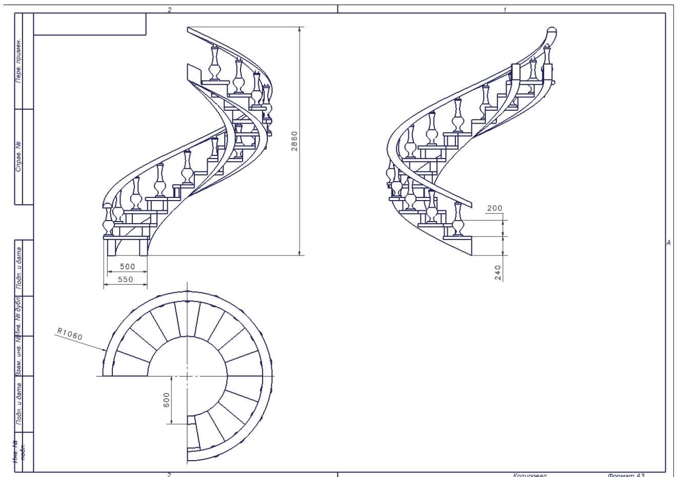
Рисунок 4 – Чертеж винтовой лестницы
